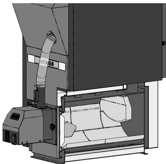
Kocioł D15PX
