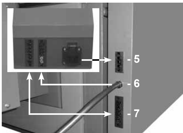
Złącza w przedniej części prawej maski kotła
