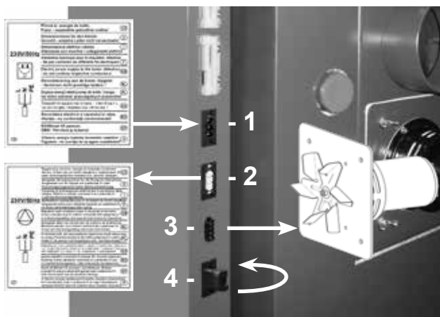
Złącza w tylnej części prawej maski kotła
